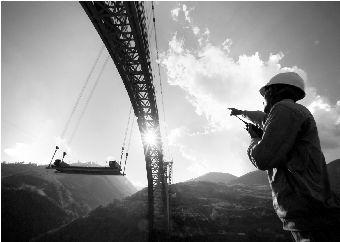
12月10日，云南大理至瑞丽铁路全线重点控制性工程——怒江四线特大桥钢桁拱顺利合龙，标志着我国“一带一路”中缅国际铁路通道建设取得重大进展。大桥主跨为单跨达490米的钢桁拱，一跨飞越怒江天堑，是目前世界上铁路拱桥的最大跨度。图为12月9日，中铁十八局技术人员指挥怒江四线特大桥钢桁杆件吊装。 新华社发（资料图片）
